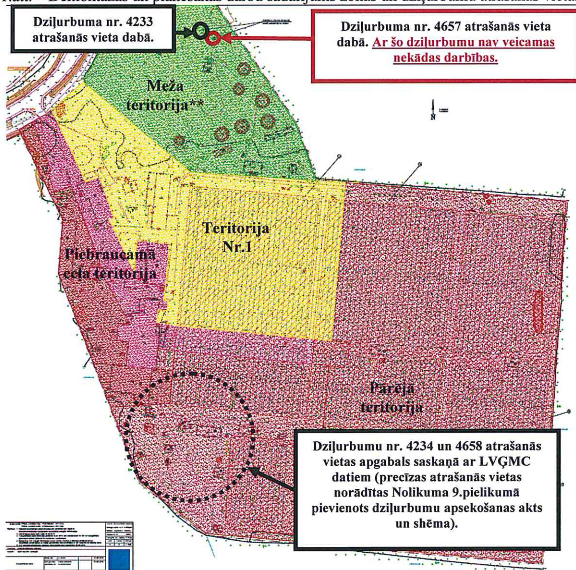
1.att. – Demontāžas un planēšanas darbu sadalījums zonās un dziļurbumu atrašanās vietas*
