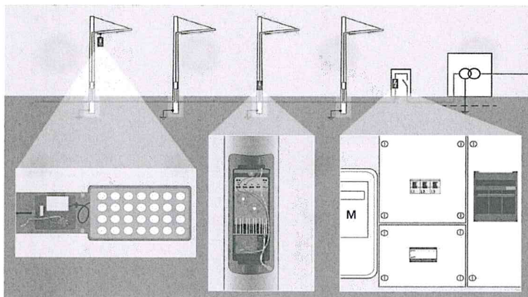
Skice Nr.2 Pārslēguma aizsardzības iespējamās uzstādīšanas vietas
