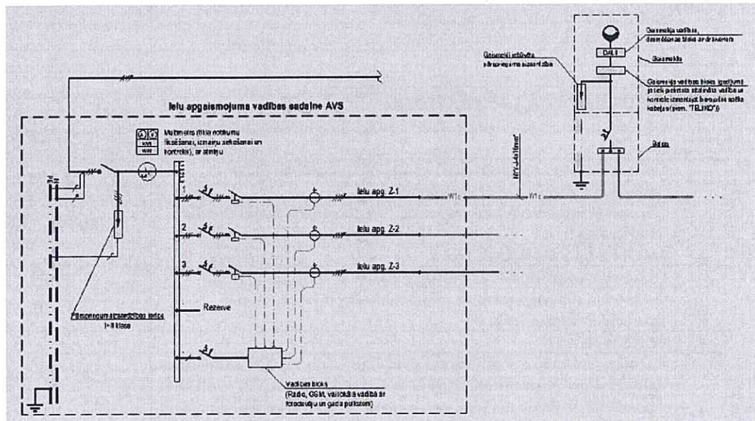
Skice Nr.1 Principāls ielu apgaismojuma shēmas risinājums
