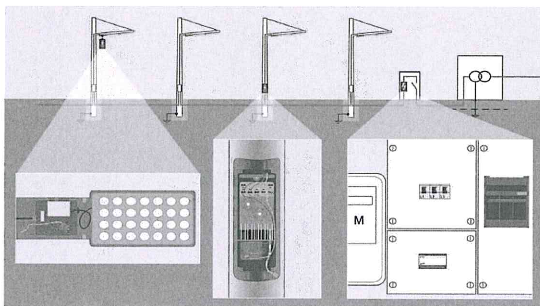
Skice Nr.2 Pārspriguma aizsardzības iespējamās uzstādīšanas vietas
