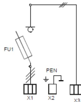
4.1.2. att. Elektriskā principshēma
