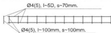
Karkass K1 (griezums un izklājums)
