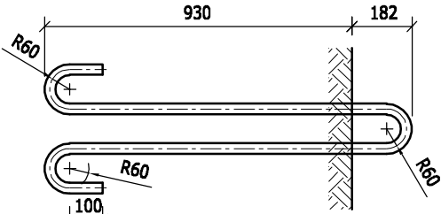
Poz.1 M 1 : 20
