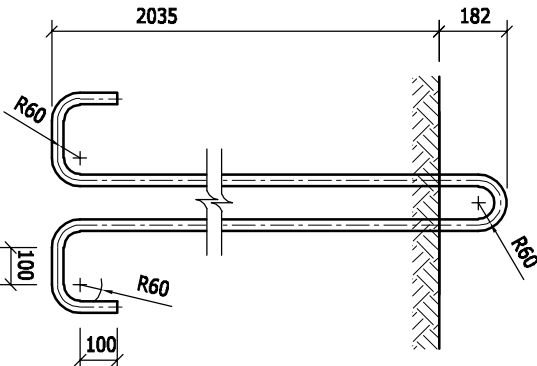
Poz.3 M 1 : 20
