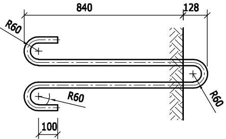
Poz.2 M 1 : 20
