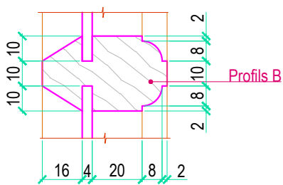
MEZGLS 2 M 1:2
