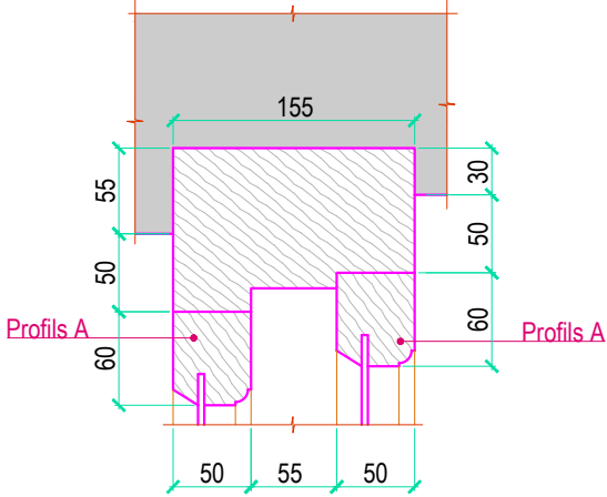
MEZGLS 3 M 1:5
