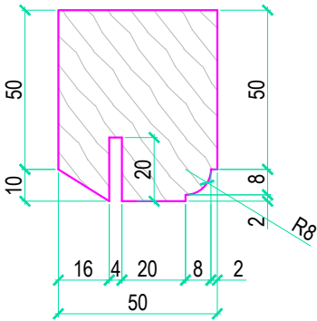
PROFILS A M 1:2
