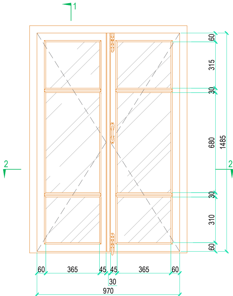
LOGA L-01 PRESTKATS (SKATS NO IEKŠPUSES) M 1:15
