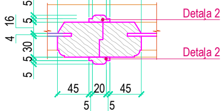
MEZGLS 4 M 1:5
