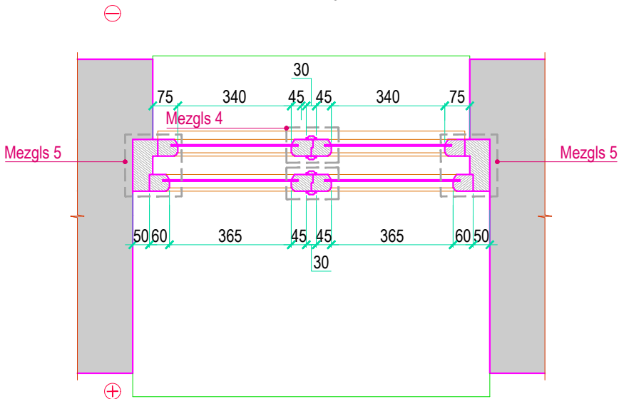
ŠKĒLUMS 2-2 M 1:15
