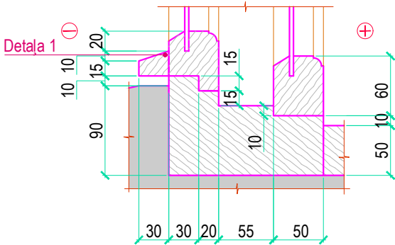
MEZGLS 4 M 1:5
