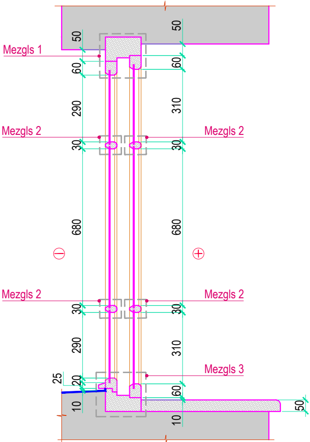
ŠKĒLUMS 1-1 M 1:15
