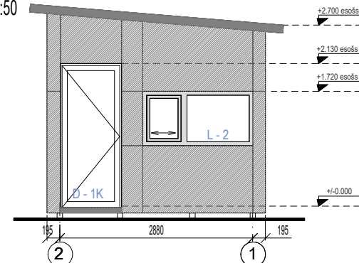
FASĀDE ASĪS A-B M 1:50
